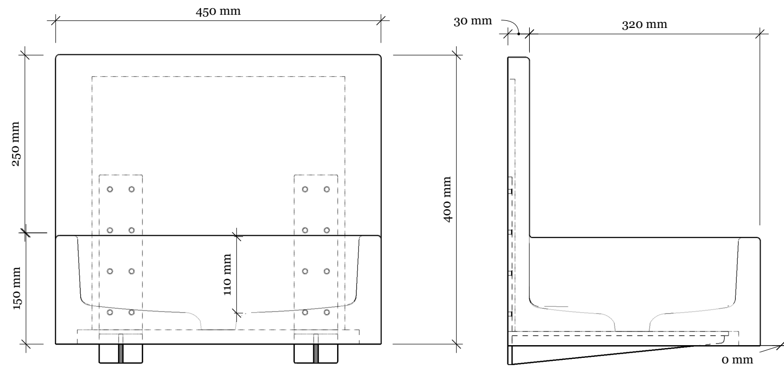
ELEVATION
