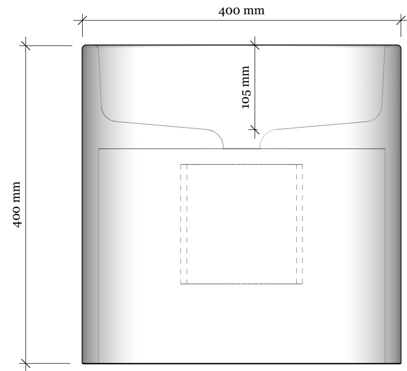
ELEVATION
